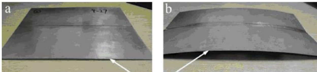
Slika 11. Savijanje [9]: a) lasersko zavarivanje b) TIG zavarivanje
