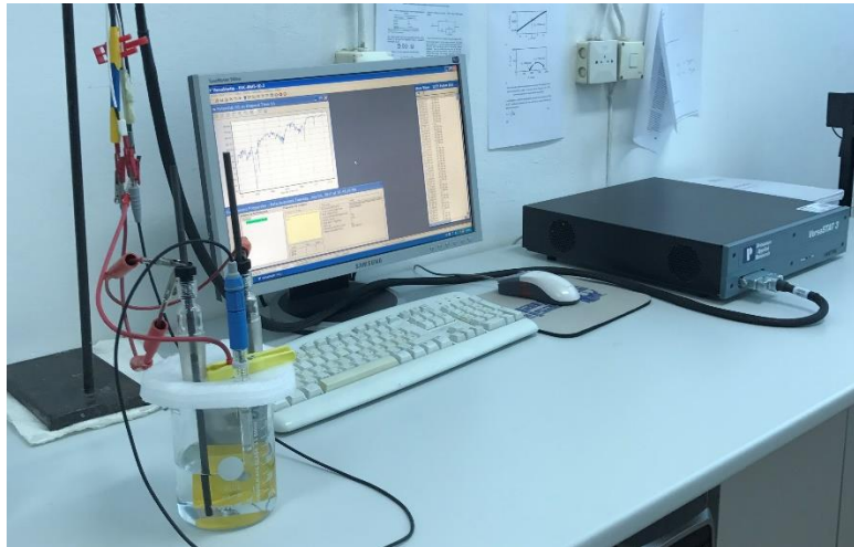
Slika 52. Oprema za ispitivanje EIS, Laboratorij za zaštitu materijala, FSB
