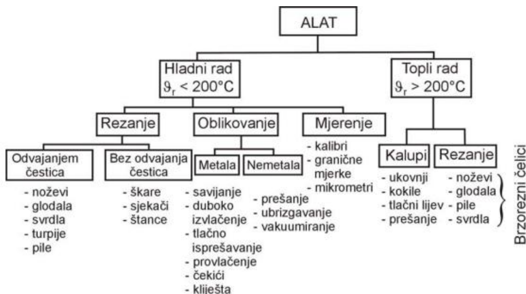
Slika 1. Podjela i primjena alatnih čelika, [1]
