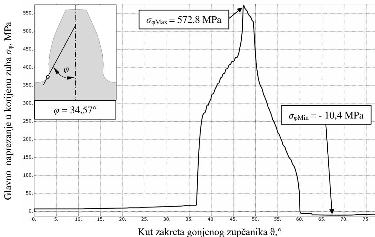
Slika 24. Ciklus napreznja korijena zuba punog zupčanika bez zarezova
