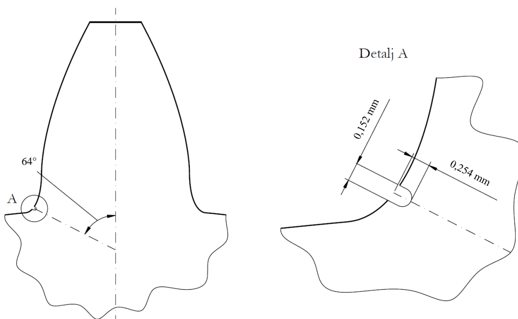
Slika 33. Dimenzije i pozicija zarezala na zupčaniku s tankim vijencem [5]
