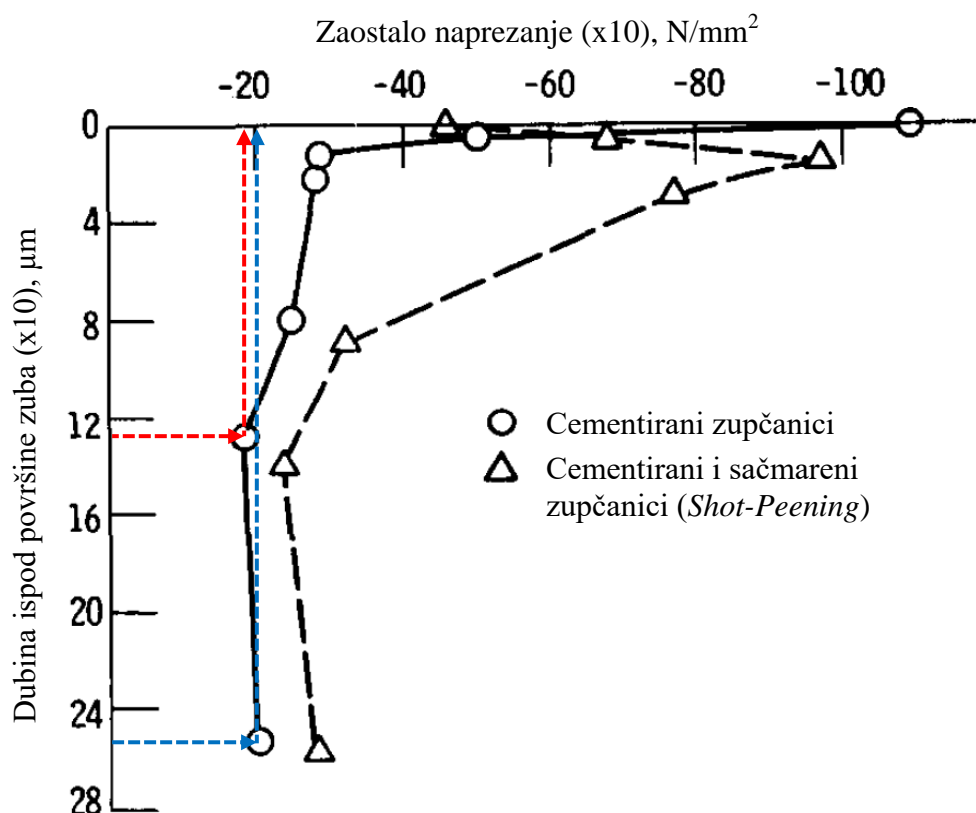
Slika 51. Prosječna vrijednost zaostalih naprezanja za cementirane i hladno očvrstute zupčanike [33]
