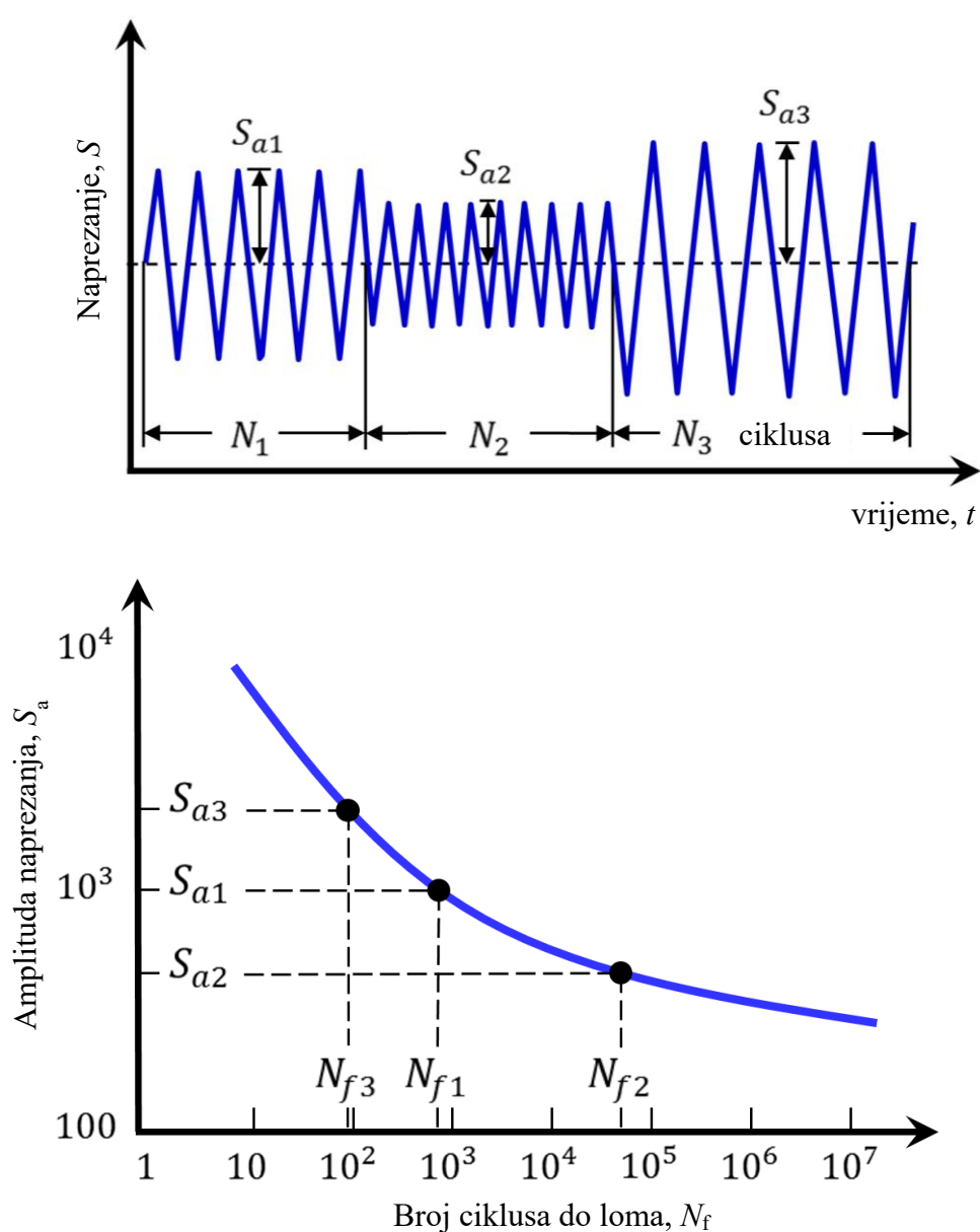
Slika 44. Palmgren-Minerovo pravilo [2]
