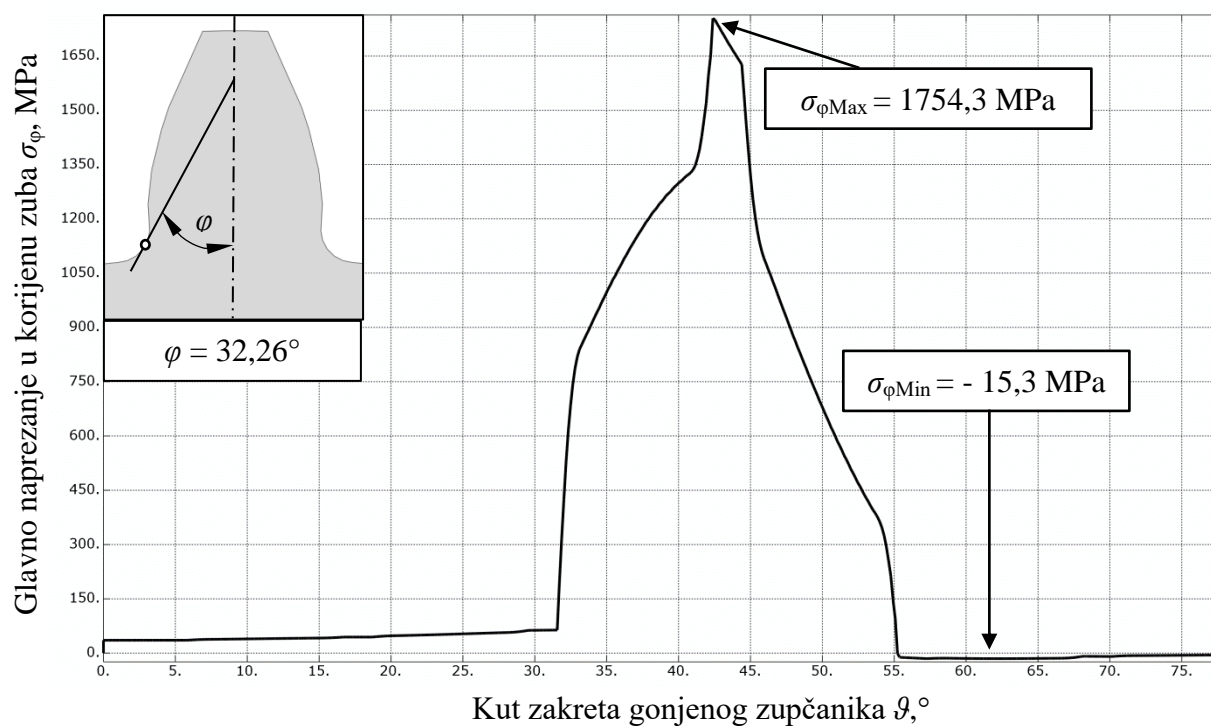
Slika 30. Ciklus napreznja korijena zuba punog zupčanika sa zarezom
