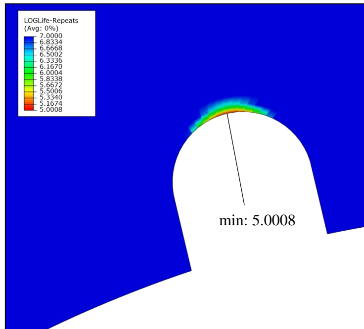
Slika 52. Kritično područje nastanka pukotine kod punog zupčanika
