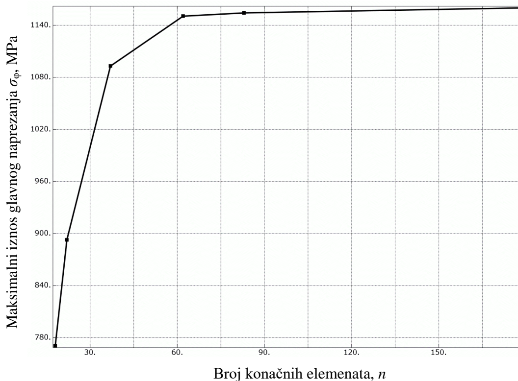
Slika 28. Konvergencija maksimalnog napreznja u korijenu zuba za slučaj 2
