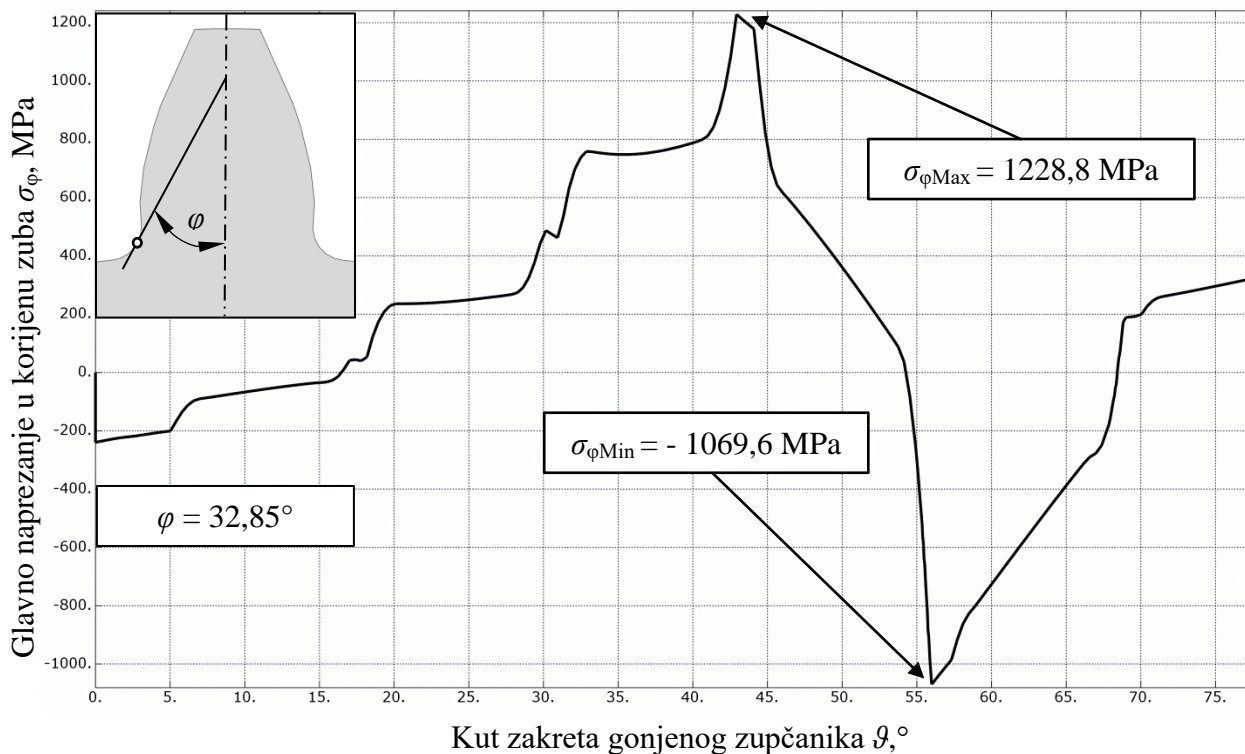
Slika 37. Ciklus napreznja korijena zuba zupčanika s tankim vijencem i zarezom
