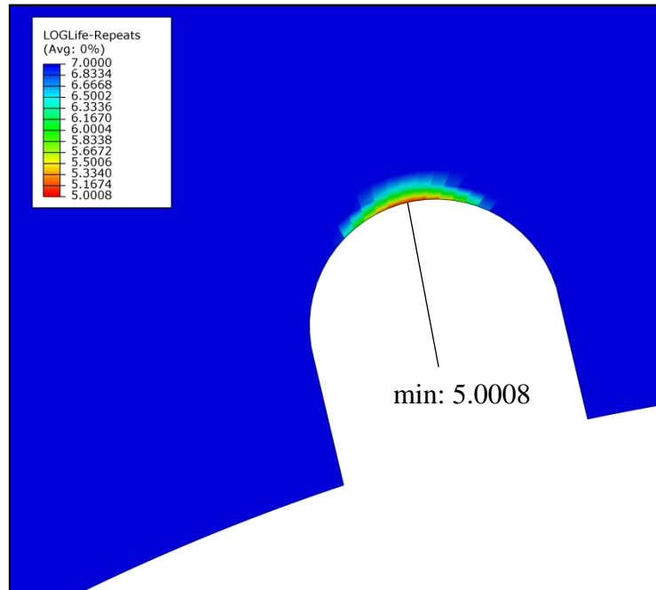
Slika 52. Kritično područje nastanka pukotine kod punog zupčanika
