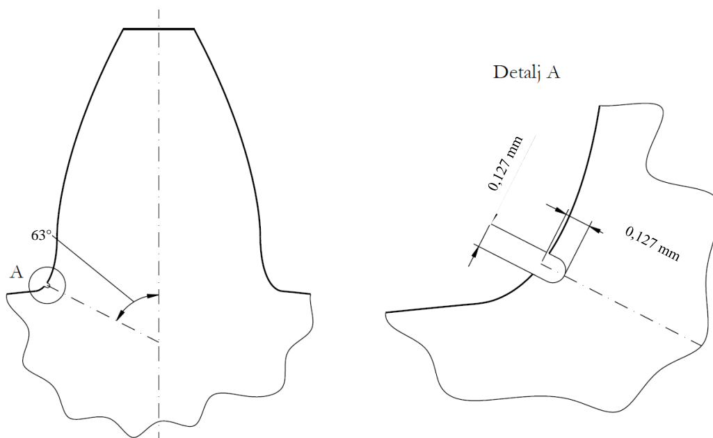
Slika 26. Dimenzije i pozicija zareza na punom zupčaniku [5]
