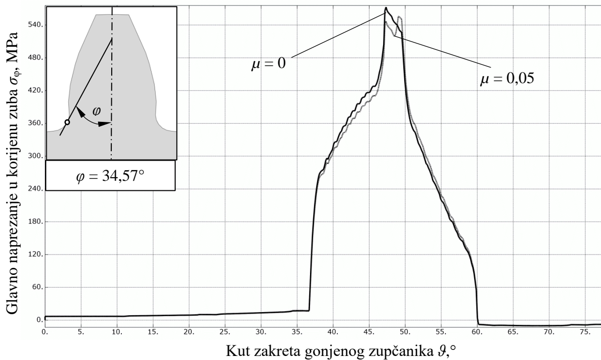
Slika 54. Utjecaj trenja na ciklus naprezanja punog zupčanika bez zarez
