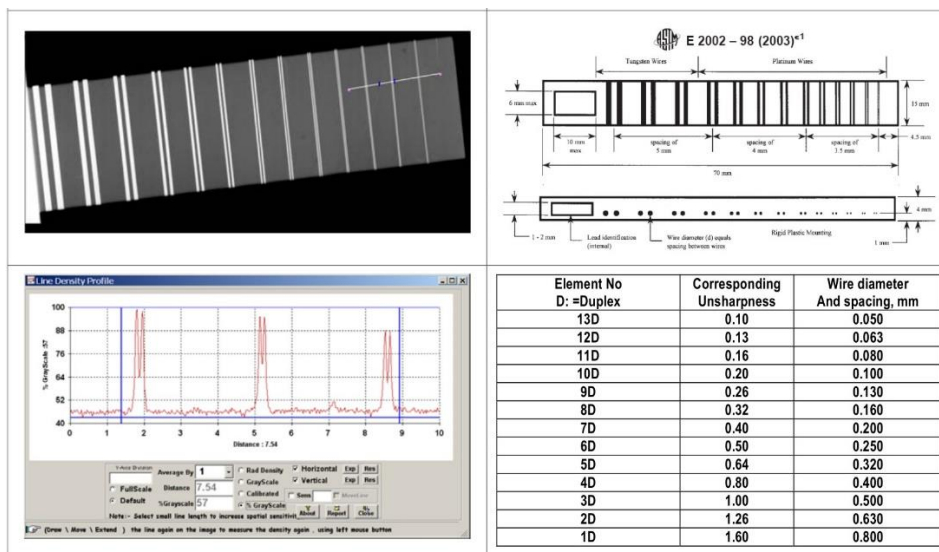
Slika 6. Duplex indikator [7]
