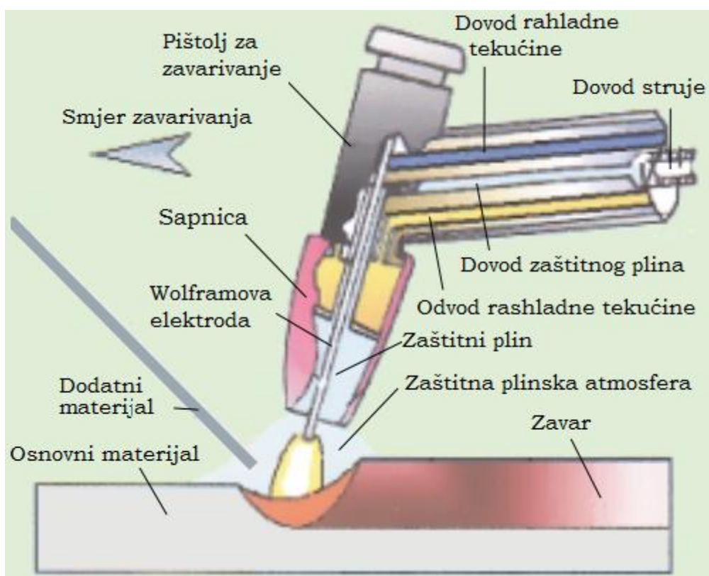
Slika 3. Schematski prikaz TIG postupka zavarivanja [8]
