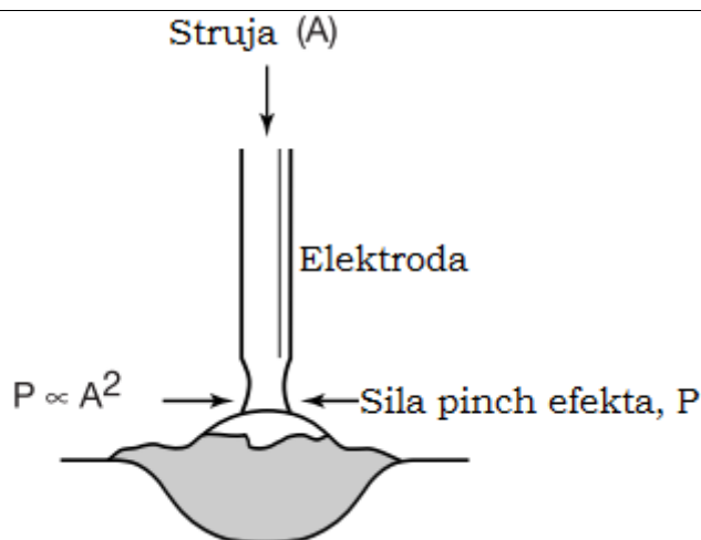
Slika 7. Shematski prikaz prijenosa metala kratkim spojevima [18]
