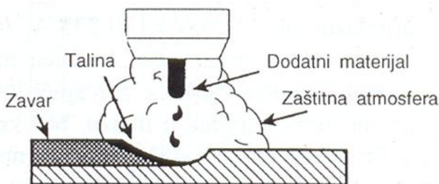
Slika 5. Shema elektrodoalnog zavarivanja taljivom metalnom elektrodom u zaštitnoj atmosferi plinova [16]
