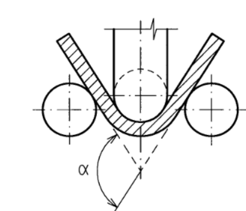
Slika 30. Prikaz ispitivanja sućeonog zavarenog spoja na savijanje [29]
