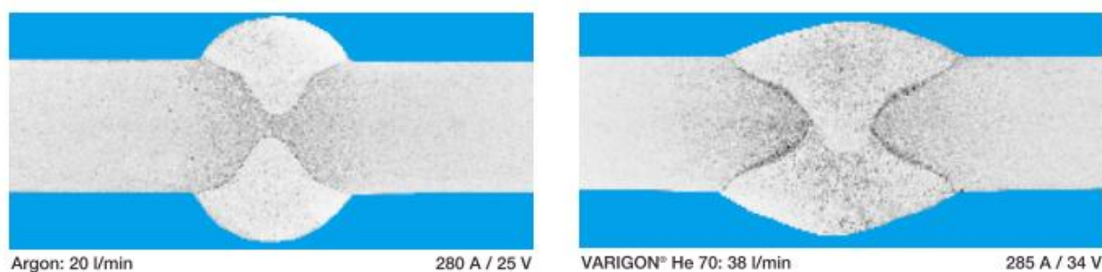
Slika 10. Usporedba utjecaja argona i helija na penetraciju i širinu zavara [19]
