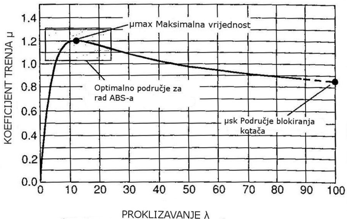
Slika 2.5 Ovisnost koeficijenta trenja o proklizavanju
