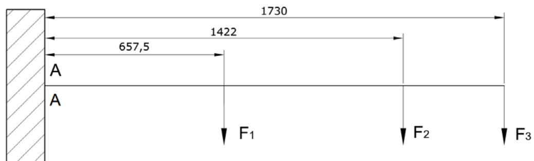
Slika 29. Opterećenje konzole
