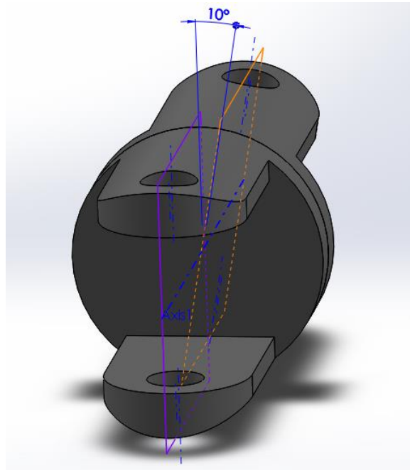
Slika 41. Otklon između vilica međuvratila
