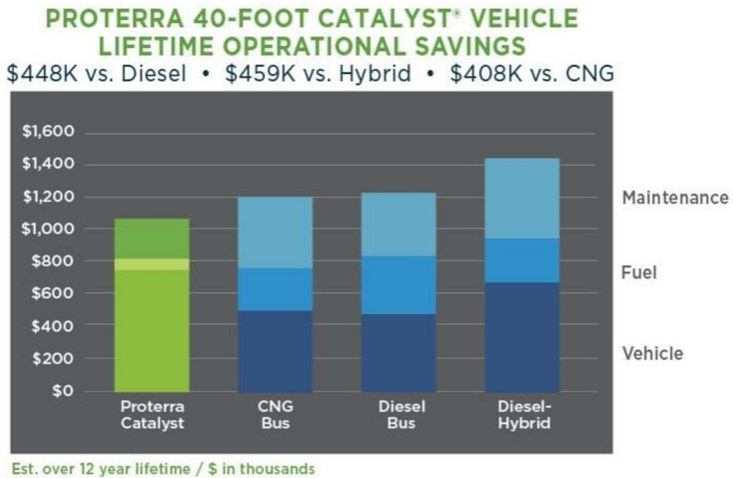
Slika 12. prikaz uštede autobusa Proterra Catalyst 40 E2 na 12-godišnjoj razini [10]
