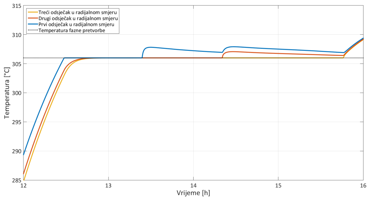
Slika 37. Detalj A – punjenje spremnika za medij u radijalnom smjeru za prvi odsječak u aksijalnom smjeru
