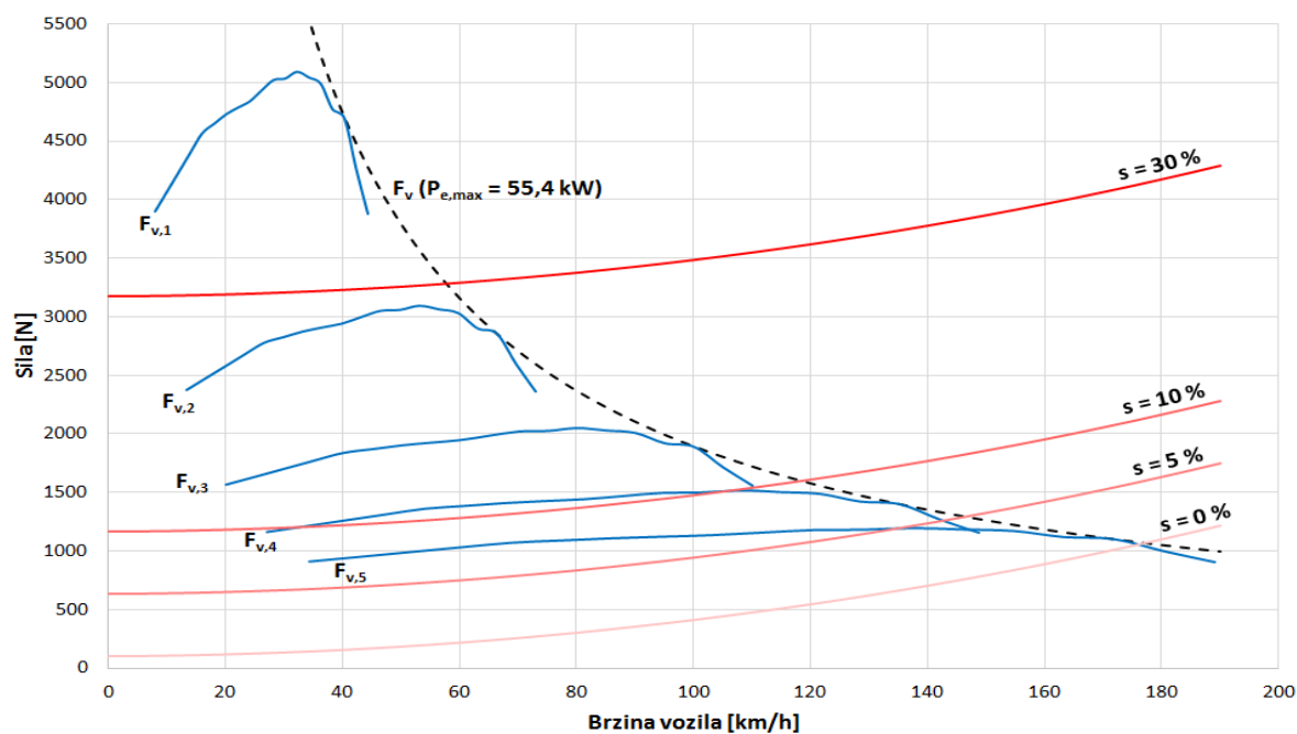
Slika 2.6. Dijagram vlačnih sila s ucrtanim otporima vožnje pri svladavanju uspona od 5, 10 i 30 %
