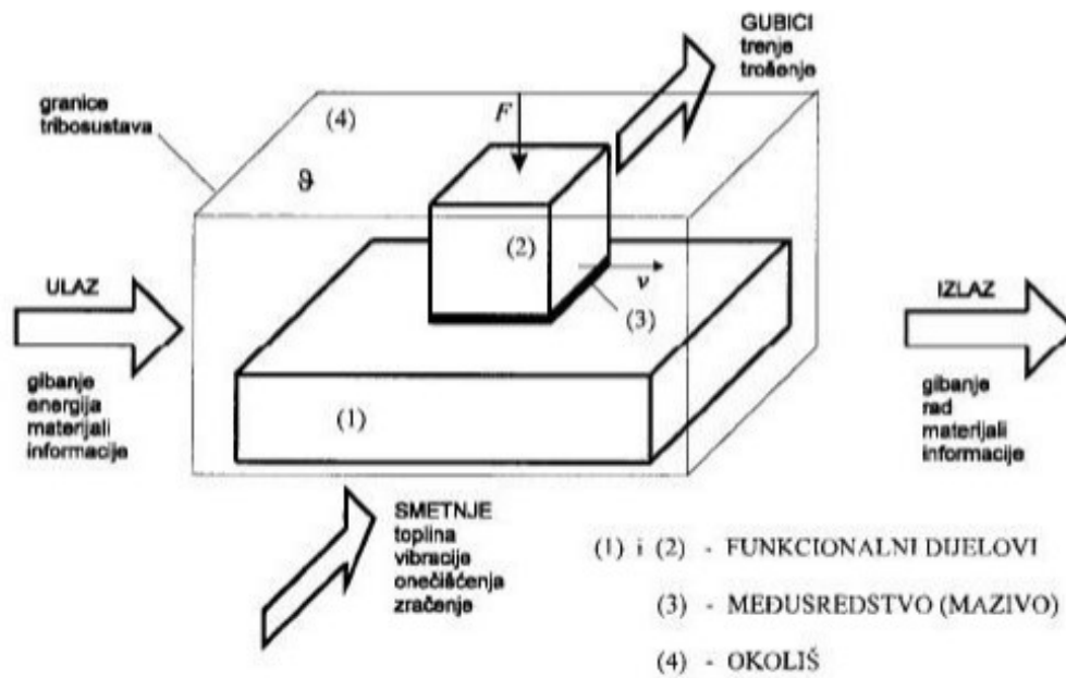
Slika 6. Osnovni tribosustav [11]
