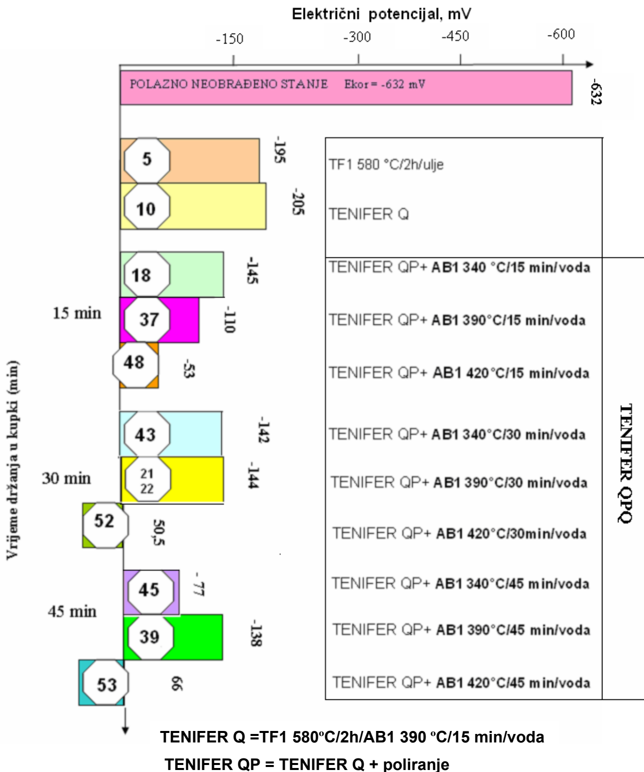
Slika 41. Utjecaj parametara naknadne oksidacije (temperature i vremena držanja na oksidativnoj kupki AB1) nitrokarburiranih uzoraka postupkom Tenifer električni potencijal pri ispitivanju korozijske postojanosti.
