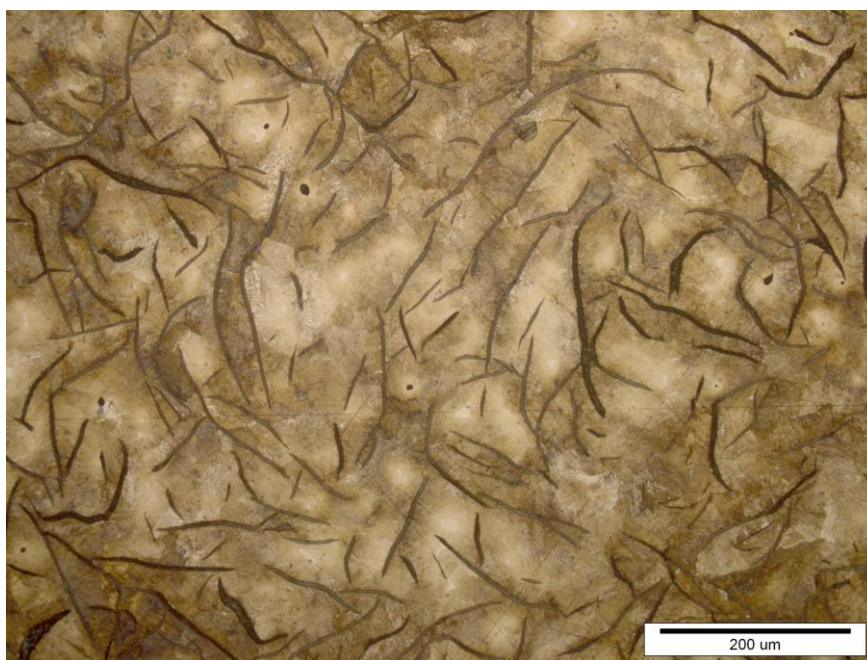
Slika 91. Mikrostruktura površine kočionog diska na svjetlosnom mikroskopu pod povećanjem 200x
