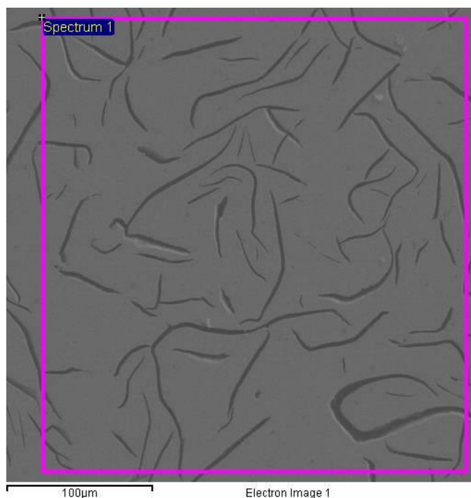
Slika 98. Područje prve analize površine uzorka kočionog diska
