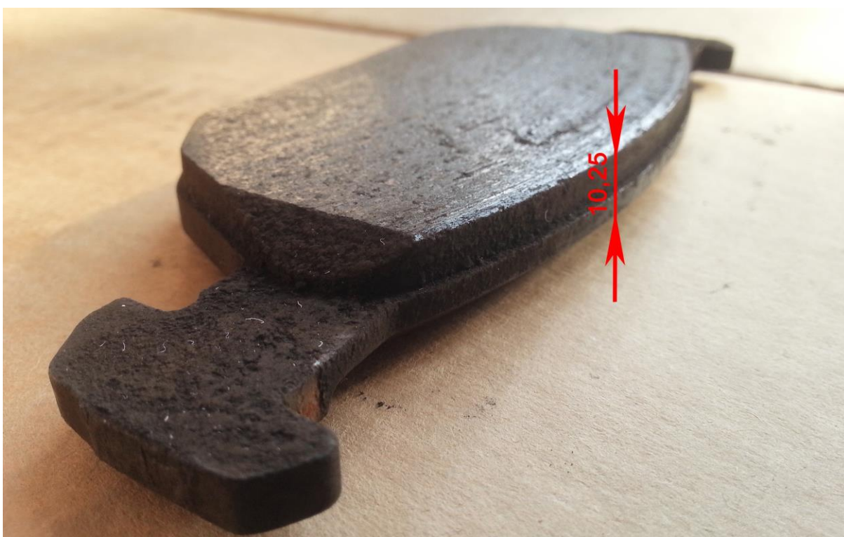
Slika 68. Debljina vanjske strane vanjske kočione pločice 1
