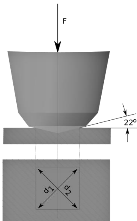
Slika 94. Skica penetratora i otiska kod metode po Vickersu
