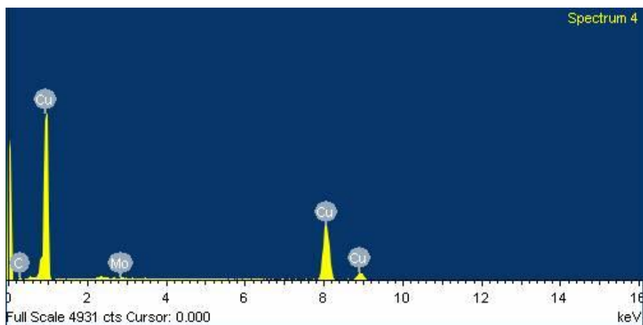
Slika 114. EDS kemijska analiza elemenata uzorka kočione obloge - 3
