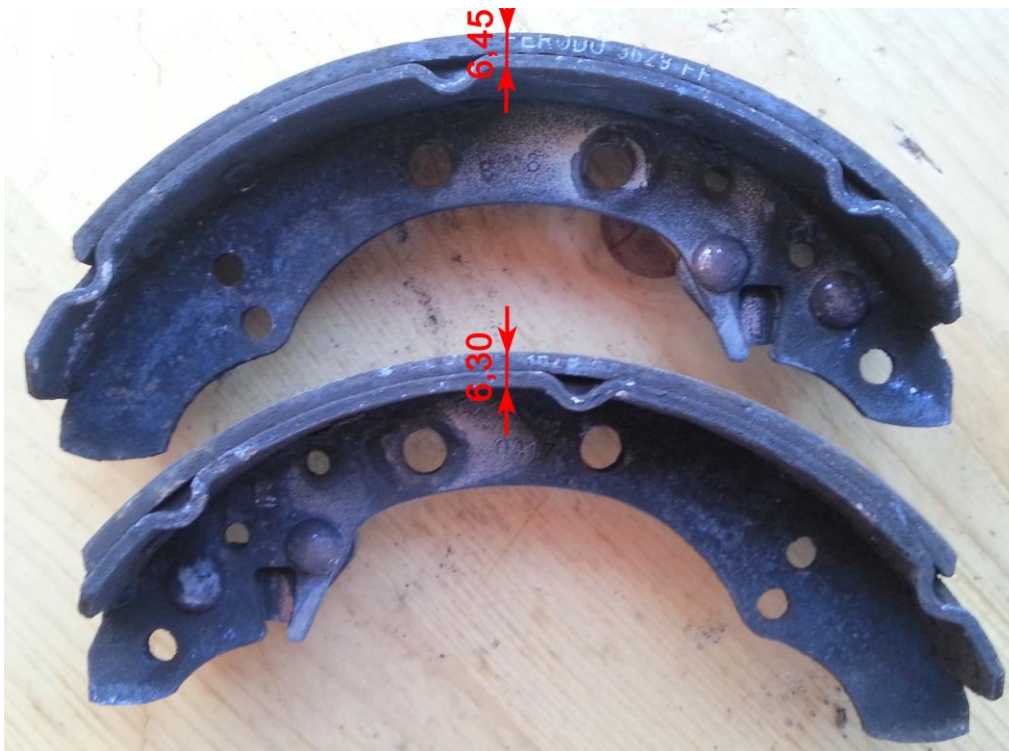
Slika 74. Debljina kočionih obloga bubanj kočnica
