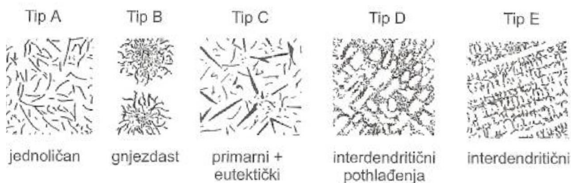
Slika 104. Tipovi listića grafita prema ASTM normi
