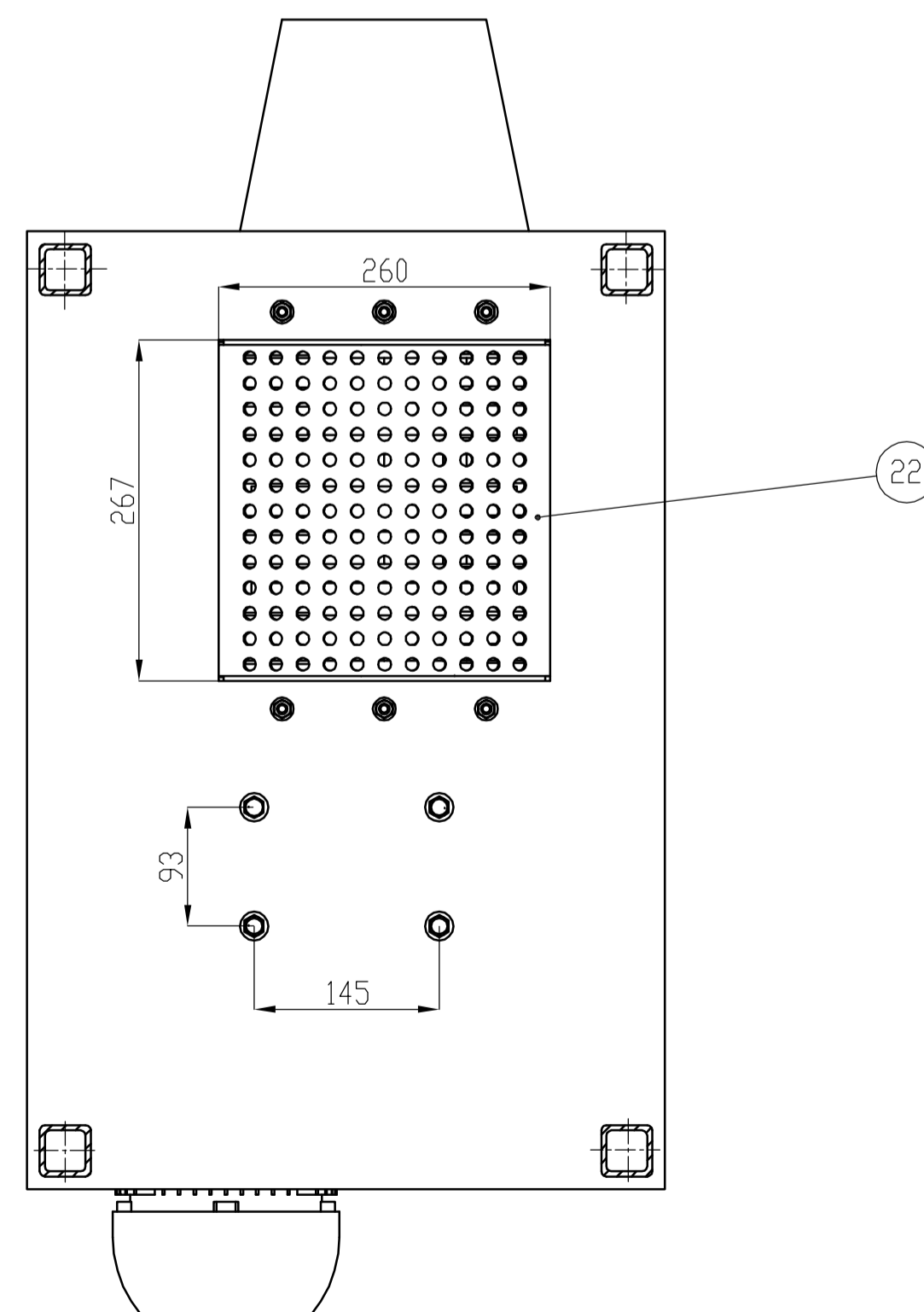
Presjek A-A M 1:5
