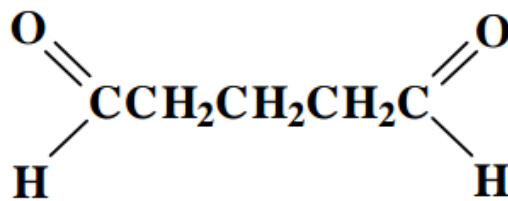
Slika 4.2 Struktura molekule glutaraldehyda (prema [37])
