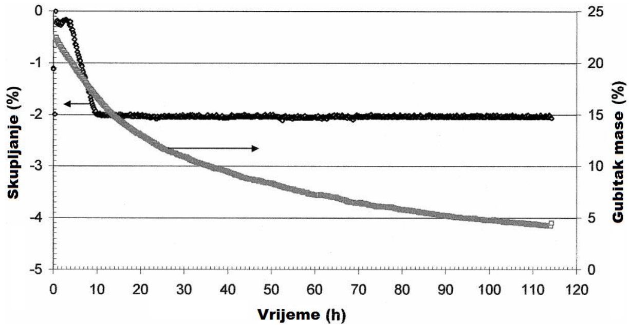
Slika 3.8 Skupljanje i gubitak mase tijekom sušenja (prema [19])
