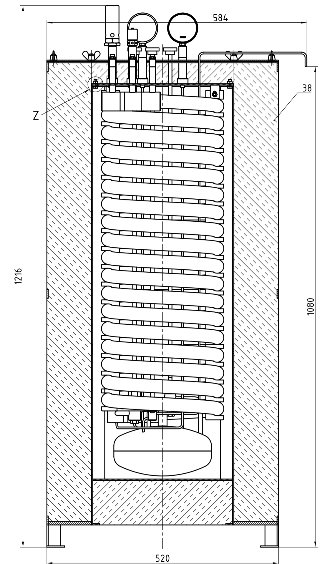
Uređaj ugrađen u izolirano kućište M 1:5
