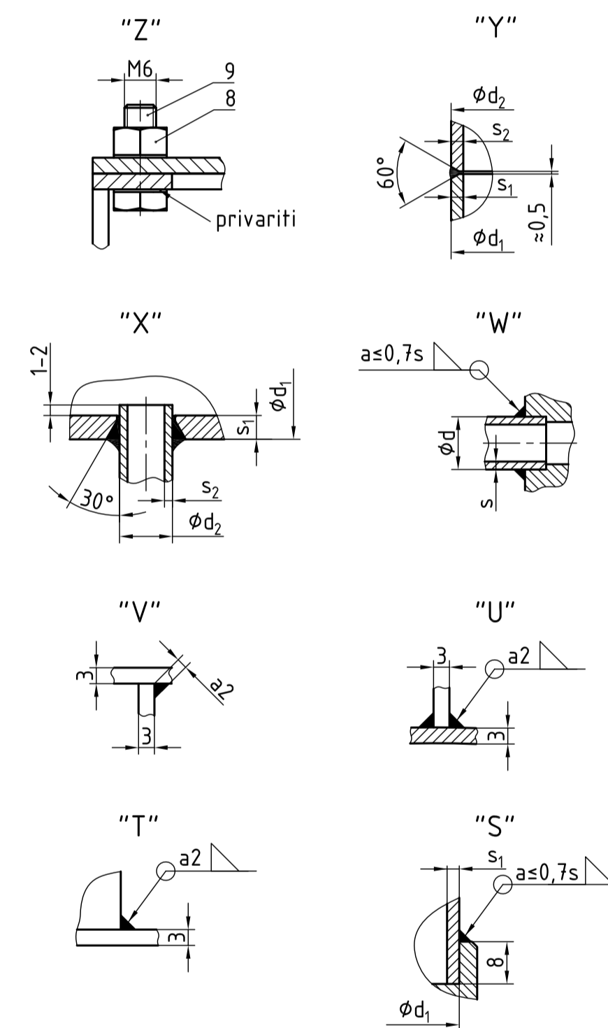
Detalji zavora M 1:1
