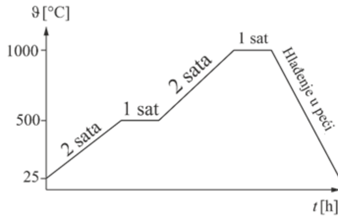
Slika 11. Dijagram toplinske obrade usitjenih ljusaka jajeta
