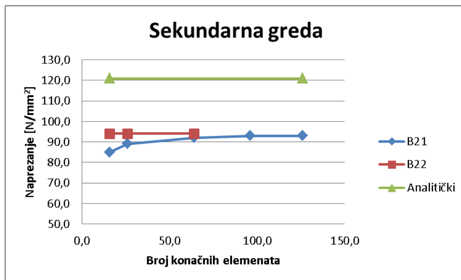
Slika 37. Sekundarna greda
