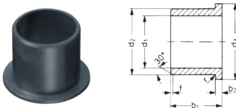
Slika 25. Ležaj s prirubnicom Iglidur H370 [12]
