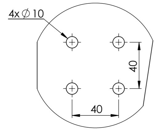
Detalj B Mjerilo (1 : 2)
