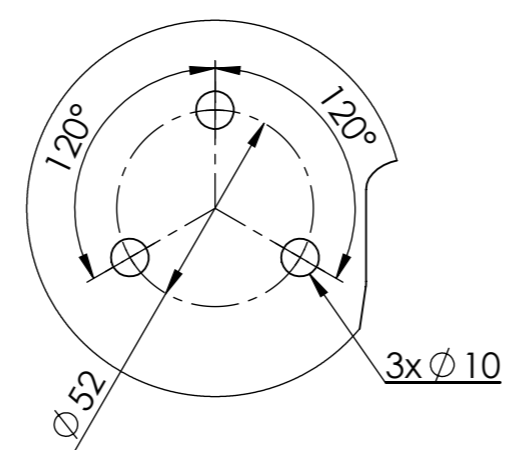
Detalj C Mjerilo (1 : 2)
