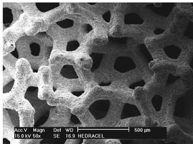
Slika 12. Porozna mikrostruktura tantala [10]
