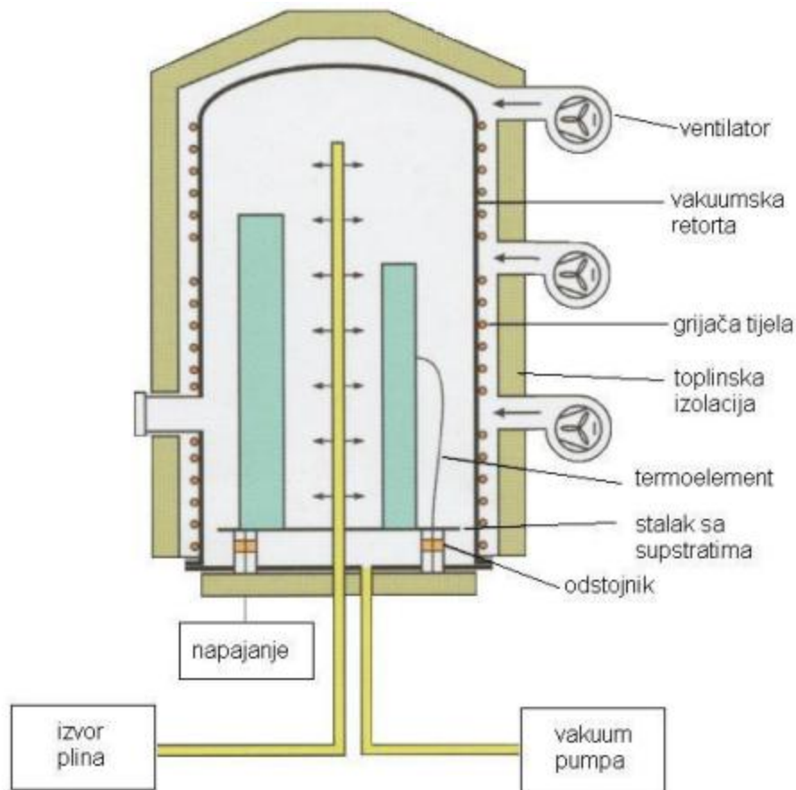
Slika 8. PACVD postupak [15]
