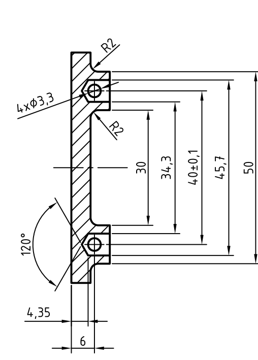
PRESJEK A-A
