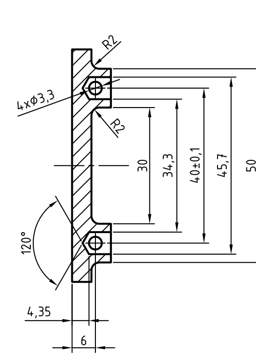
PRESJEK A-A
