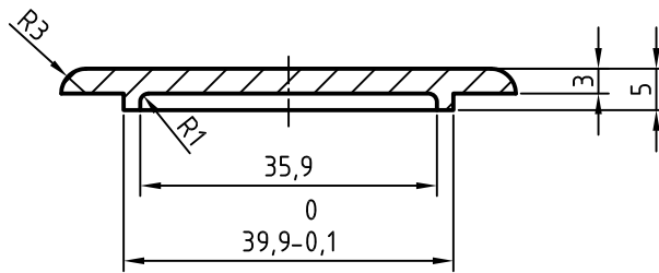
PRESJEK A-A
