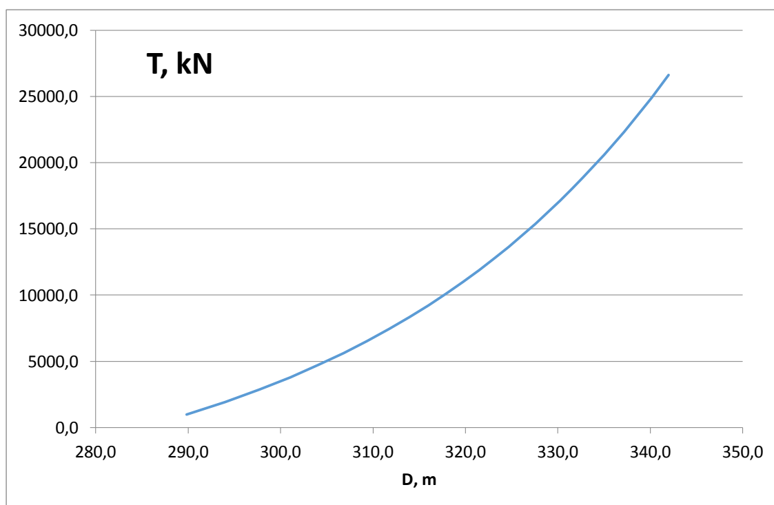
Slika 22. Ovisnost tlačne sile o horizontalnom pomaku hvatišta za T=22\text{m}
