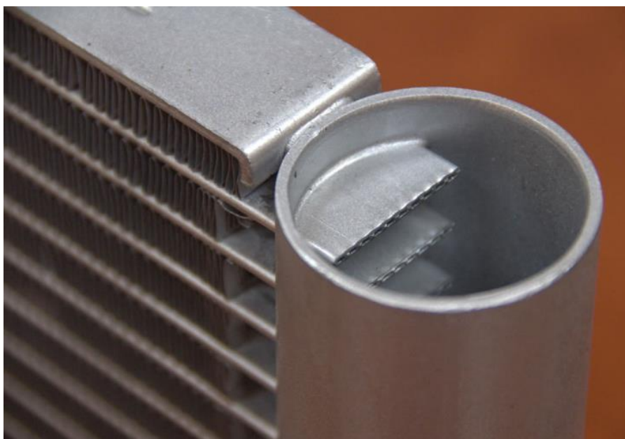
Slika 18. Detalj prikaza ravne cijevi s više usporednih mikrokanala [24]
