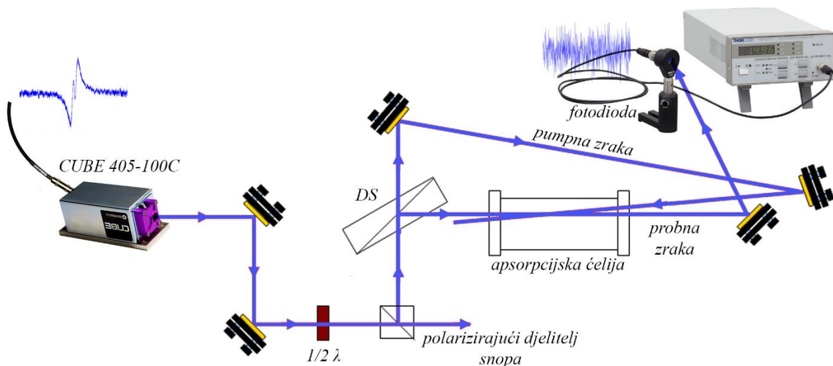
Slika 70. Postav stabilizacije CUBE 405-100C lasera
