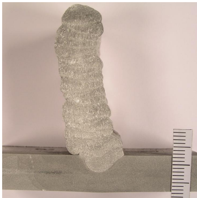
Slika 44. Makroanaliza uzorka 2
