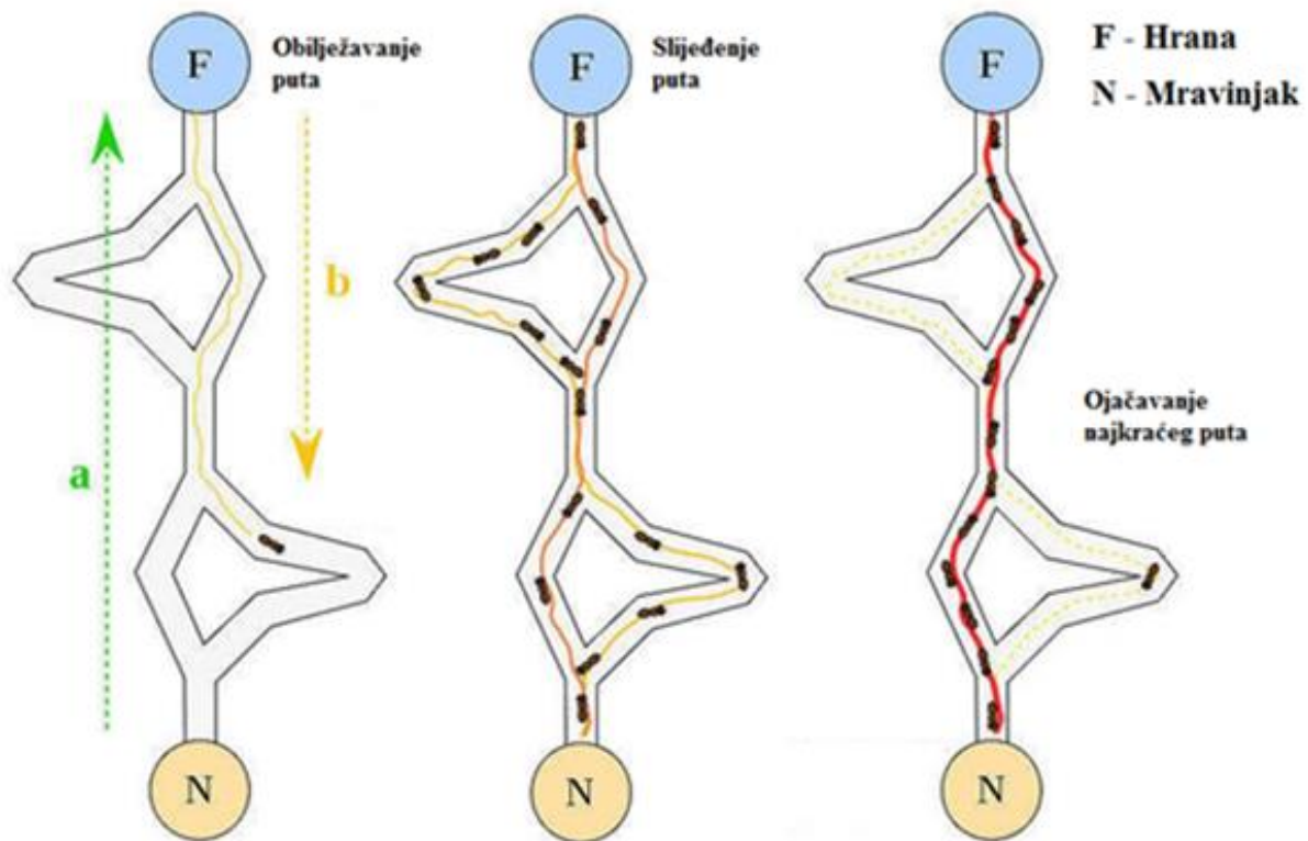
Slika 4.6 Eksperiment ACO-a [21]
