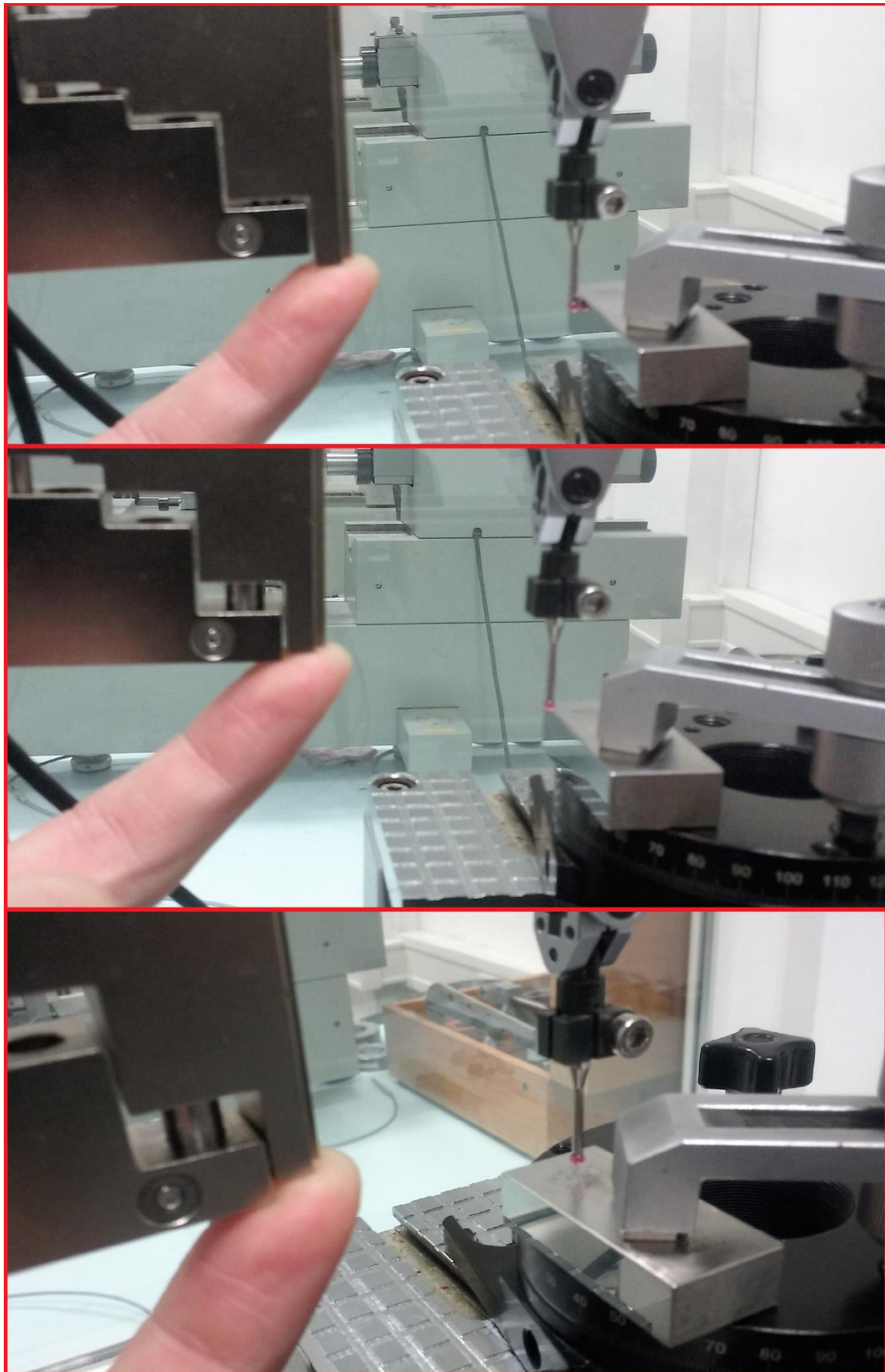
Slika 55. Translacija ticala
