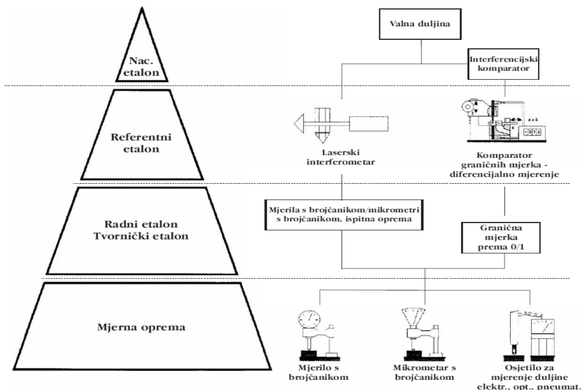
Slika 4. Hijerarhija etalona
