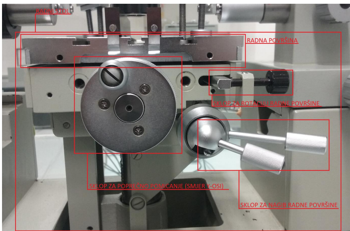
Slika 25. Radni stol
