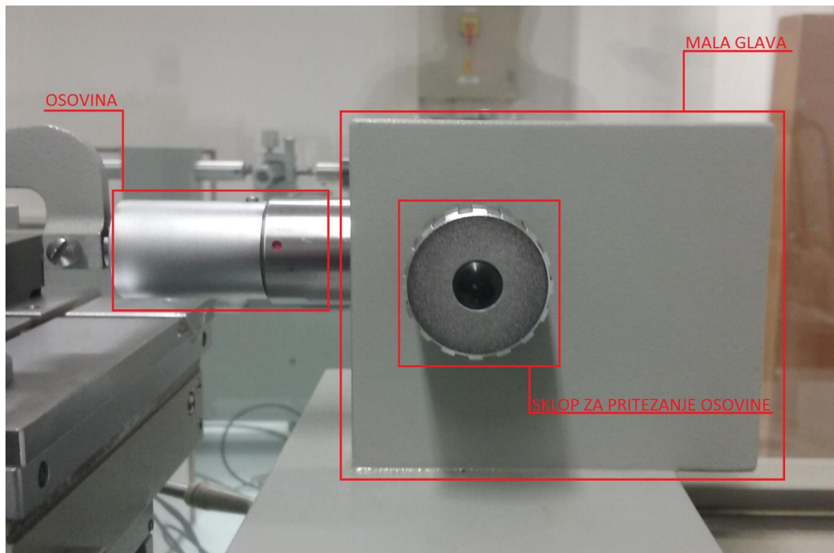
Slika 24. Mala glava
