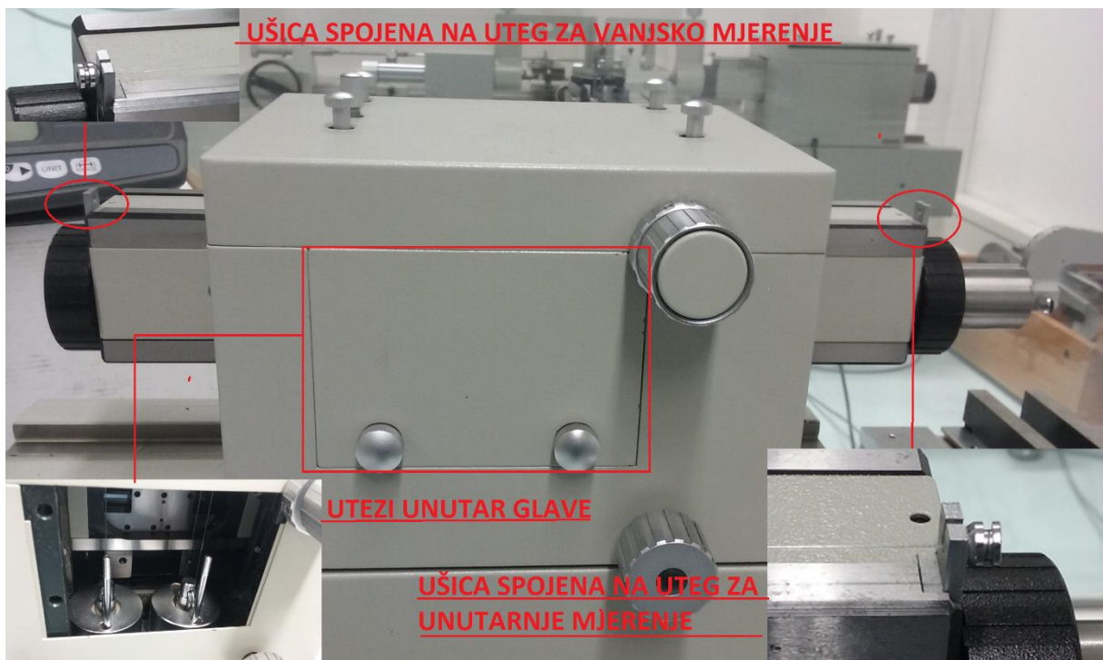
Slika 34. Pričvršćivanje ušice
