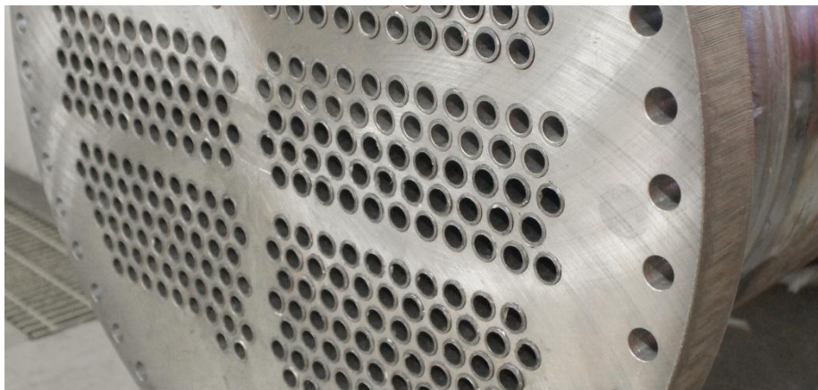
Slika 8. Spoj cijevi s cijevnom stijenom [10]
