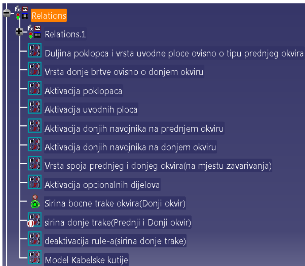
Slika 7.44 Pravila modela
