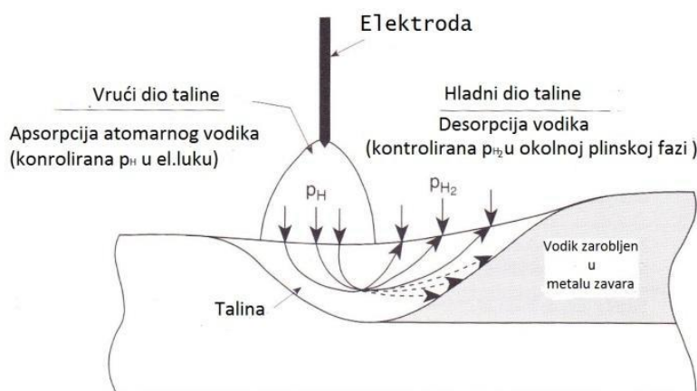
Slika 18. Mehanizam apsorpcije vodika [13]
