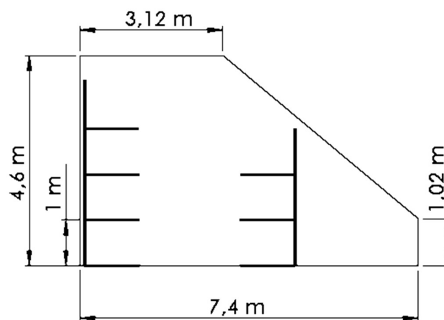
Slika 43. Peta varijanta – sirovine – presjek
