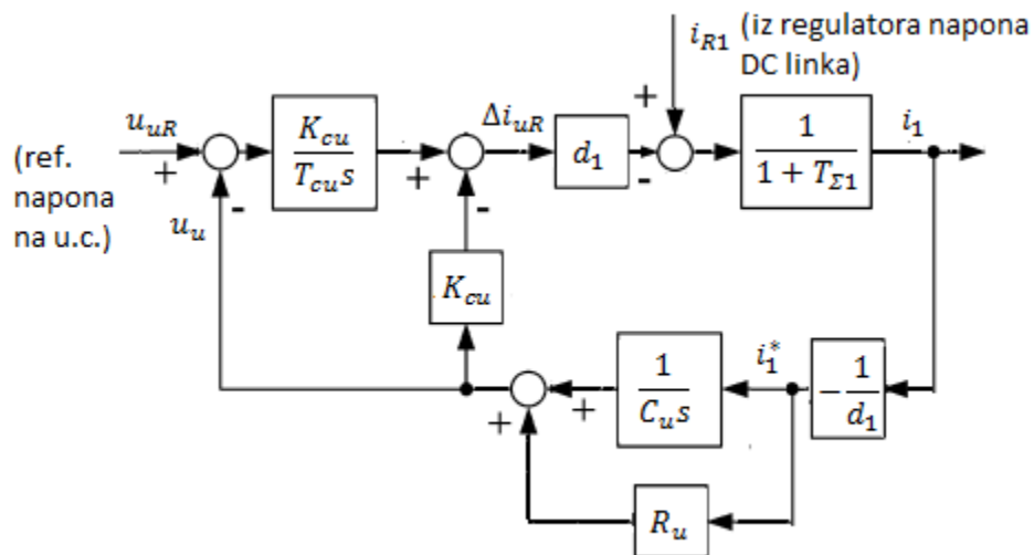
Slika 33 Struktura regulacijskog kruga SoC regulatora ultrakondezatora
