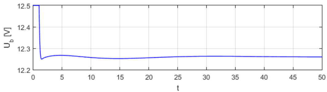
Slika 34 Odziv izlaznog napona DC sabirnice
