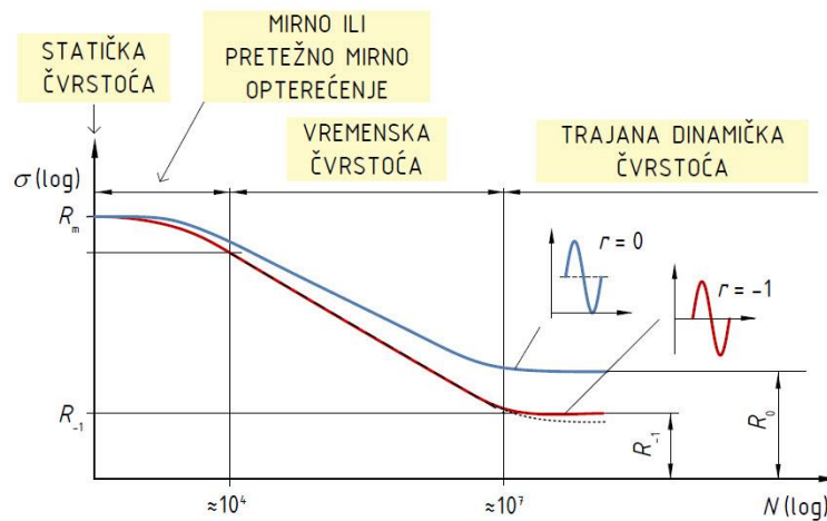
Slika 7. Wöhlerov dijagram
