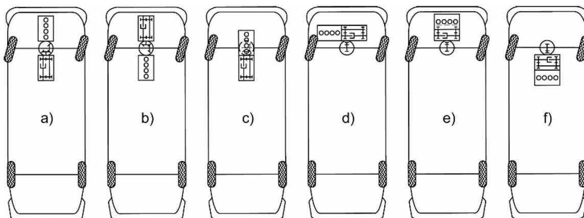
Slika 1 Konfiguracije pogona na prednje kotače
