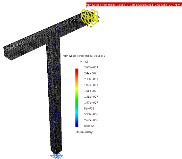
Slika 4: Puni profil - raspodjela napreznjanja kad na postolje djeluje samo jedan robot
