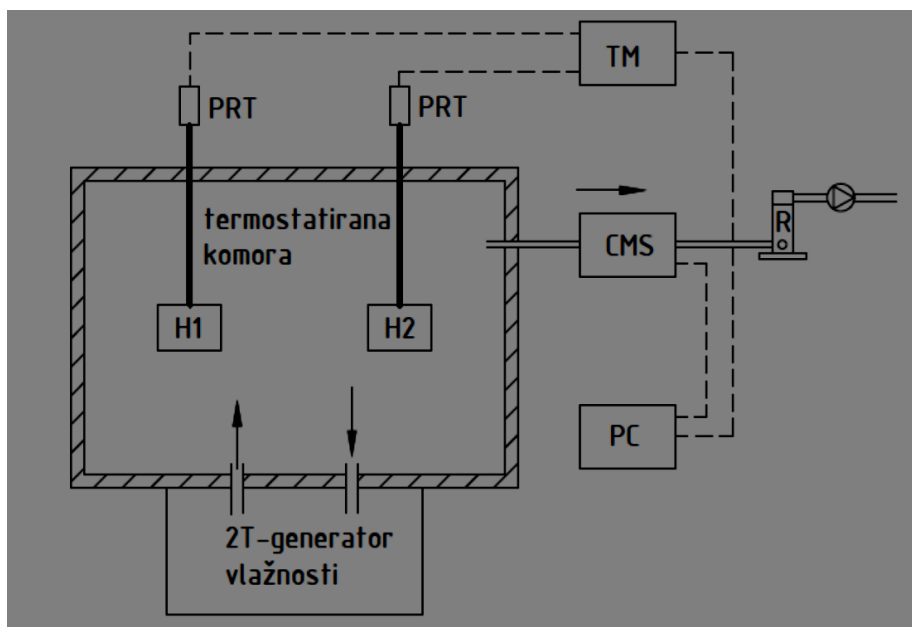
Slika 12. Komora za umjeravanje s mjerenjem temperature točke rose i ispitne temperature
