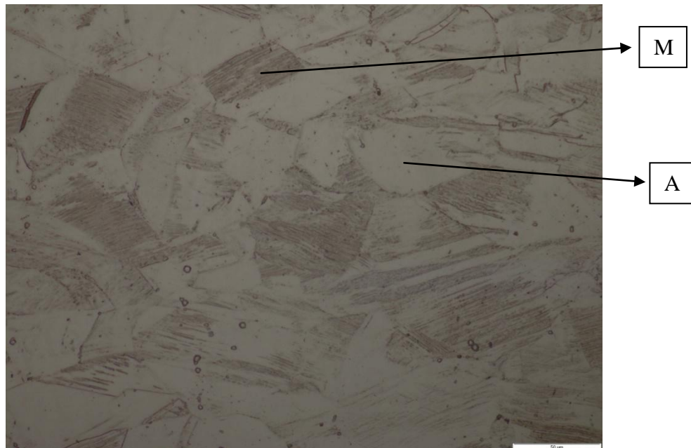
Slika 23. Mikrostruktura (A+M)
