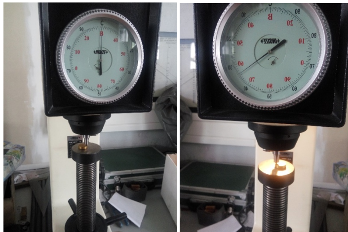
Slika 18. Ispitivanje adhezivnosti na Rockwell-owom tvrdomjeru
