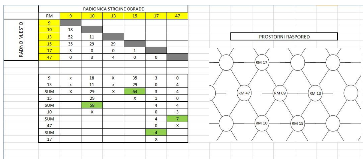
Slika 16. Modificirana metoda trokuta – jedan odjel
