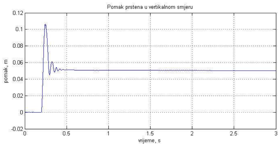
Slika 37. Vertikalni pomak prstena
