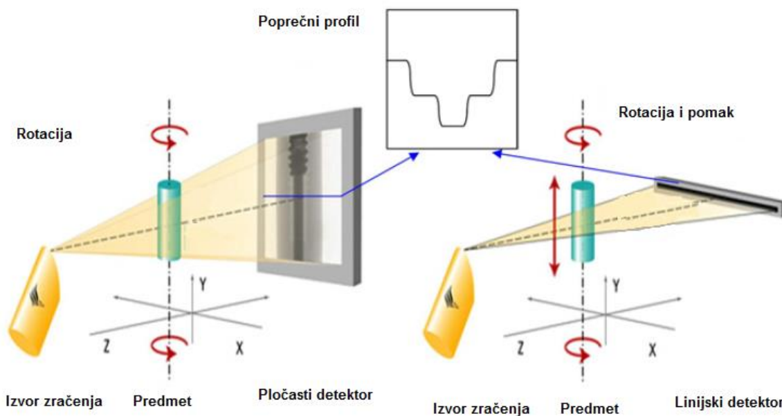
Slika 9. Vrste detektora [2]
