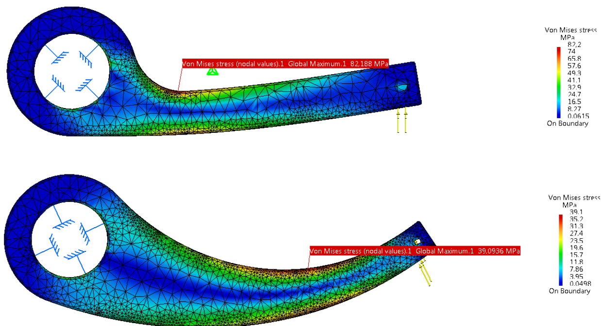
Slika 8.35. Rezultati simulacije
