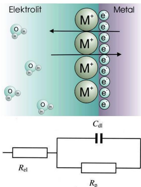
Slika 20. Randlesov krug [20]
