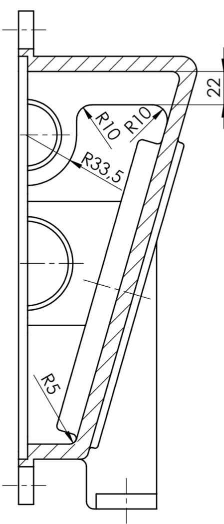
PRESJEK B-B
