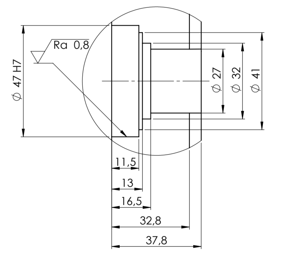
DETALJ D (1 : 1)
