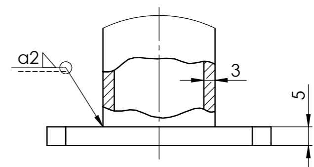
DETALJ C (1 : 1)
