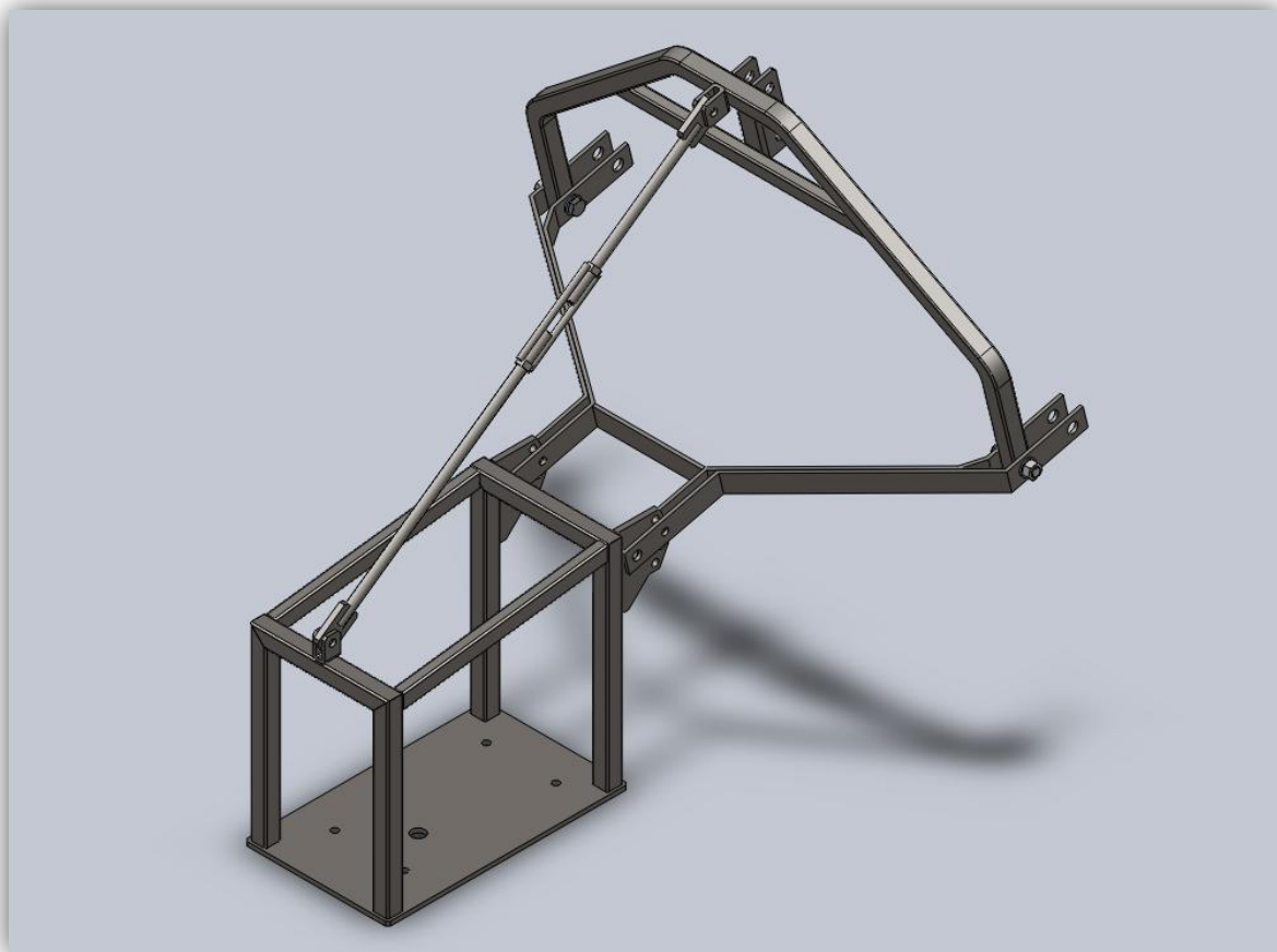
Slika 75. Nosiva konstrukcija i trotočni prihvata
