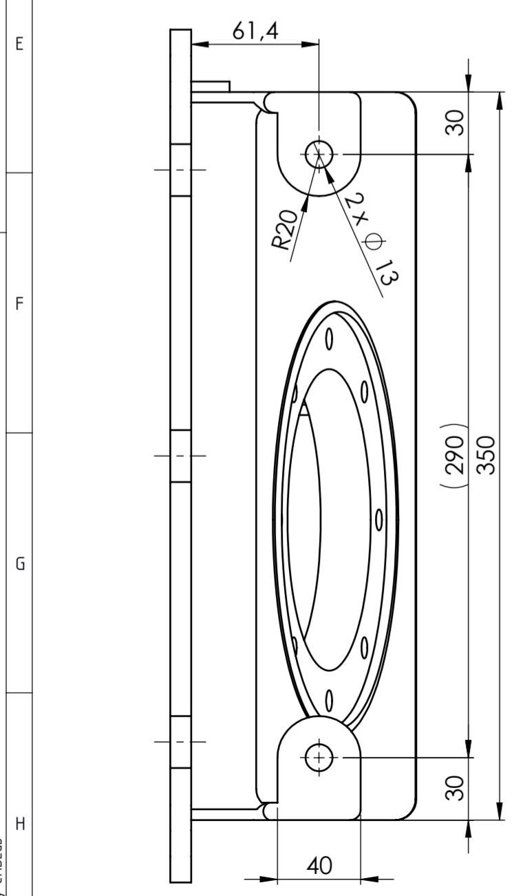
PRESJEK A-A
