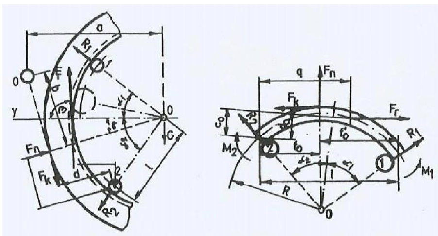
Slika 30. Sile na iskapački rotor A
