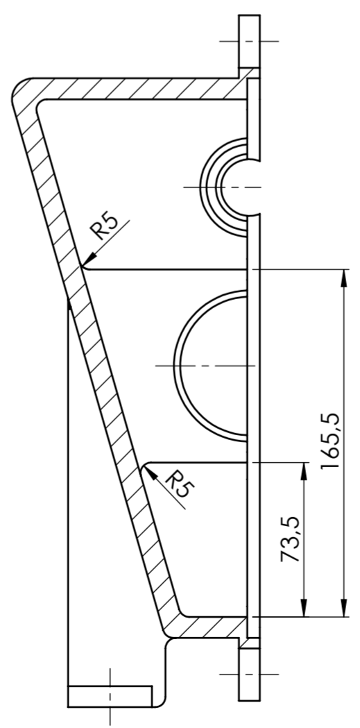
PRESJEK C-C
