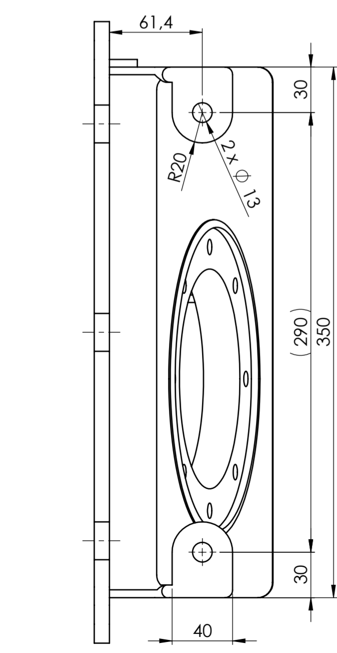
PRESJEK A-A
