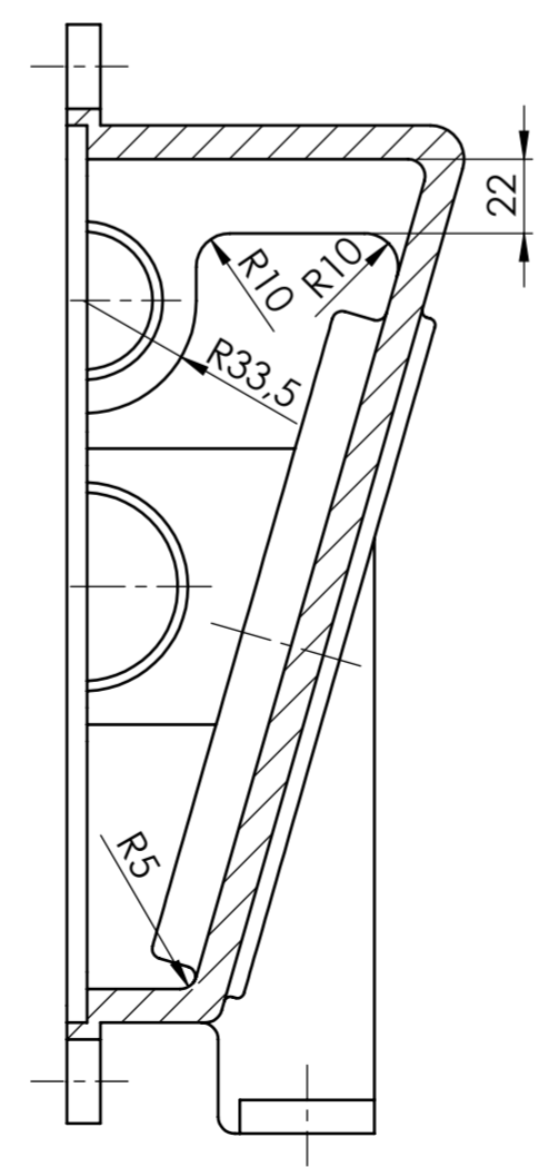
PRESJEK B-B
