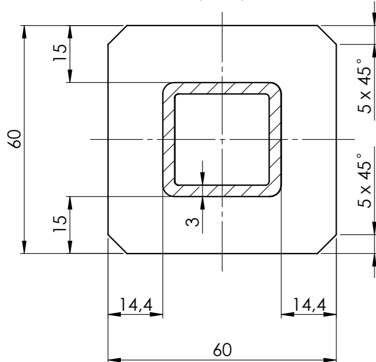
PRESJEK A-A (2 : 1)
