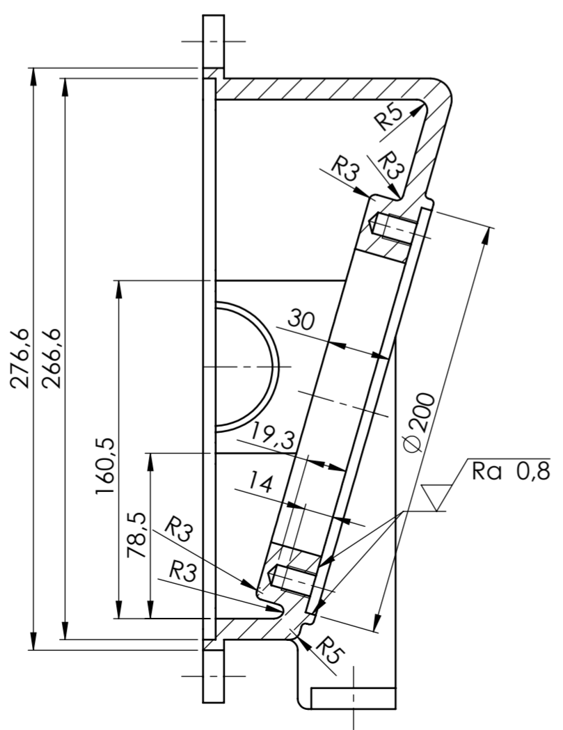
PRESJEK A-A
