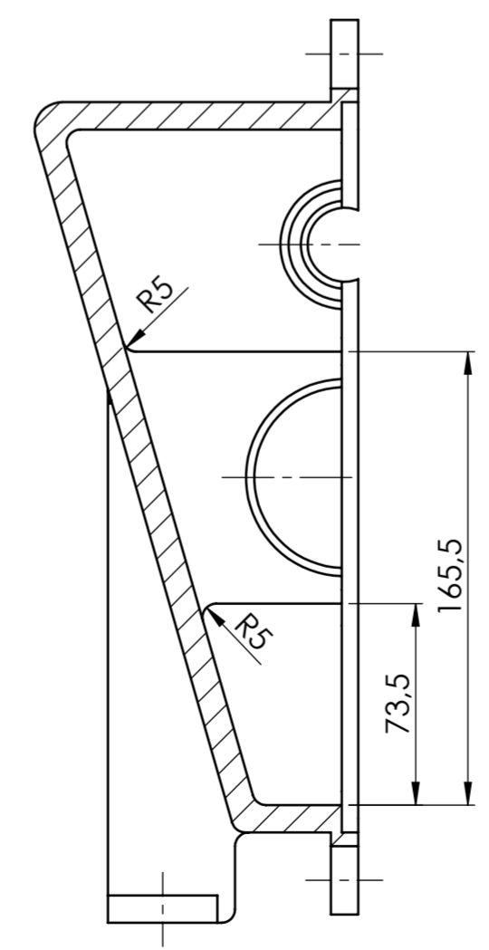
PRESJEK C-C
