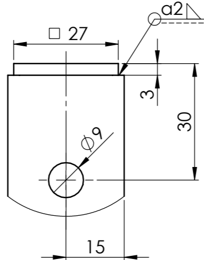
DETALJ B (1 : 1)
