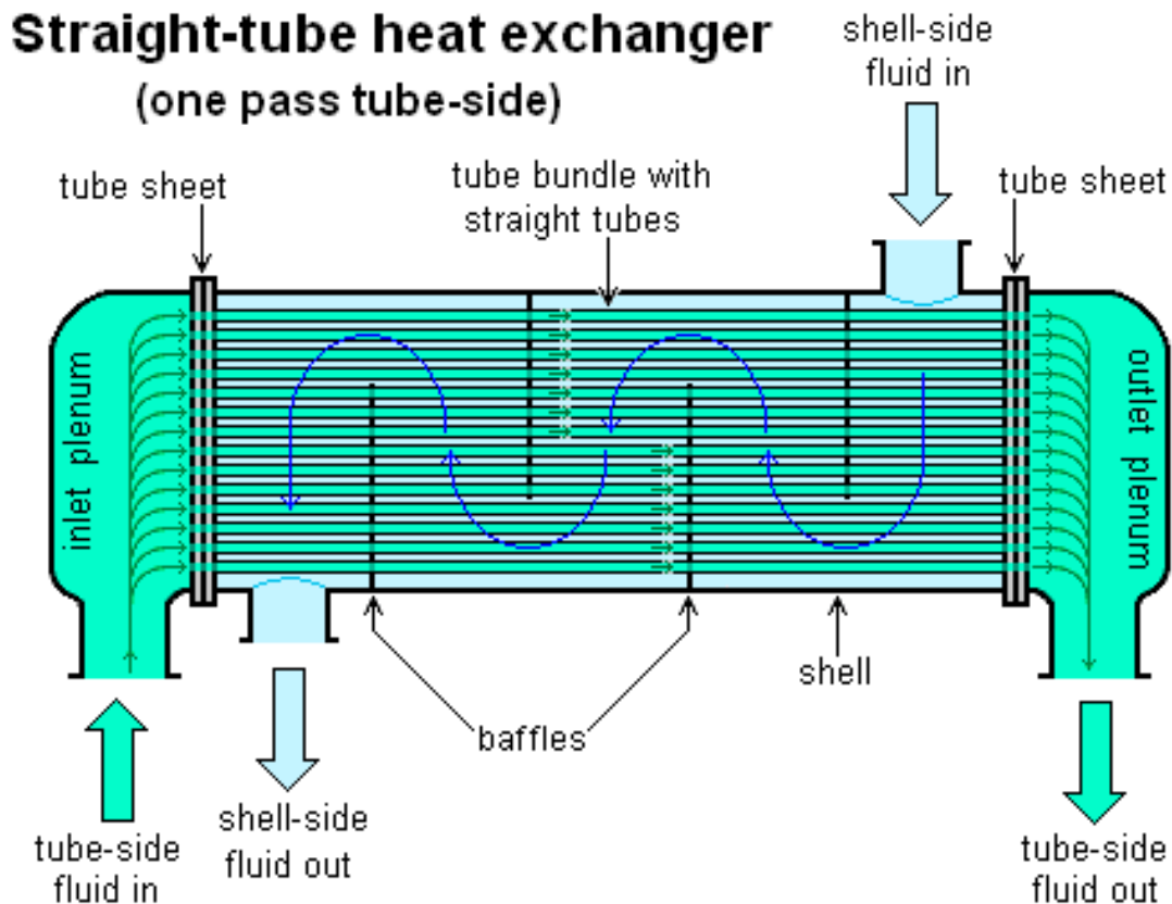
Slika 57. Izmjenjivač topline
