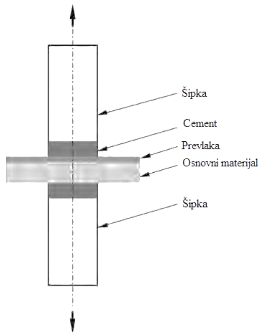
Slika 25. Test vučenja [12]
