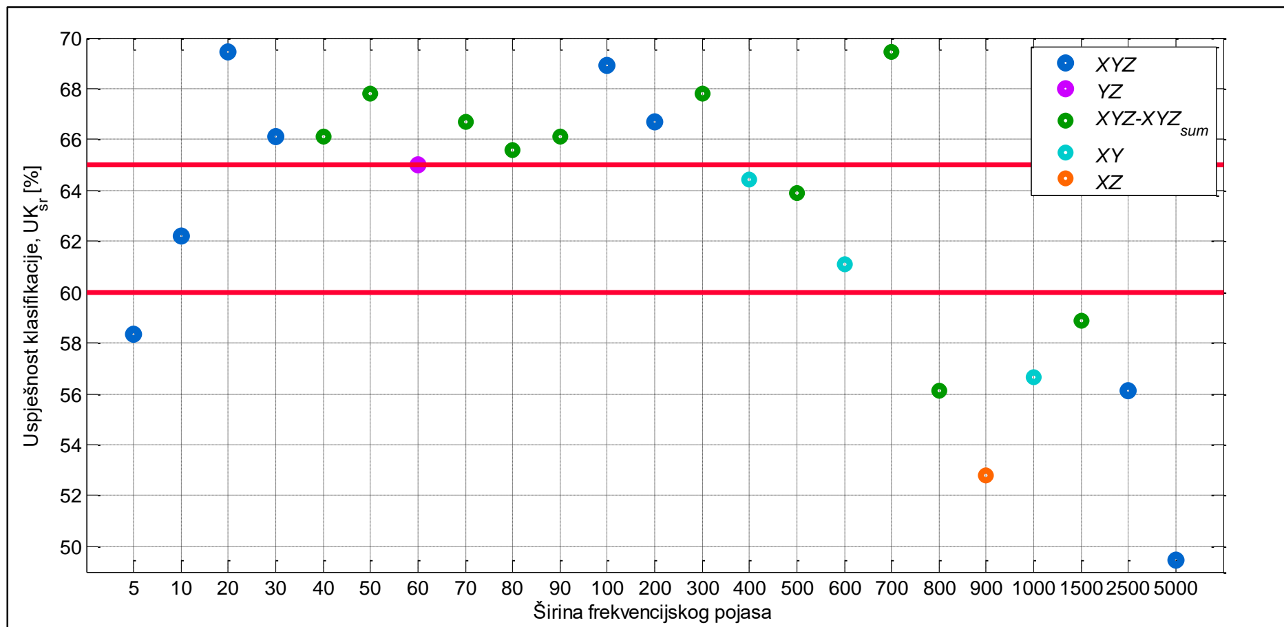
Slika 24. Najbolji rezultati analize signala vibracija za svaku širinu frekvencijskog pojasa uz Gaussovu AF i coef = 2
