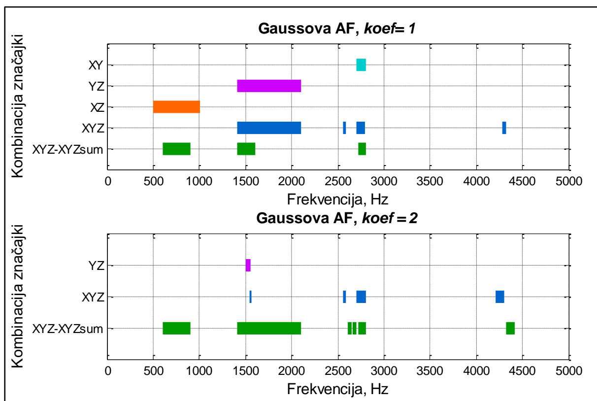
Slika 29. Odabrani frekvenzijski pojasevi za kombinacije značajki signala vibracija koje su ostvarile UK_{sr} \geq 65\% uz Gaussovu aktivacijsku funkciju
