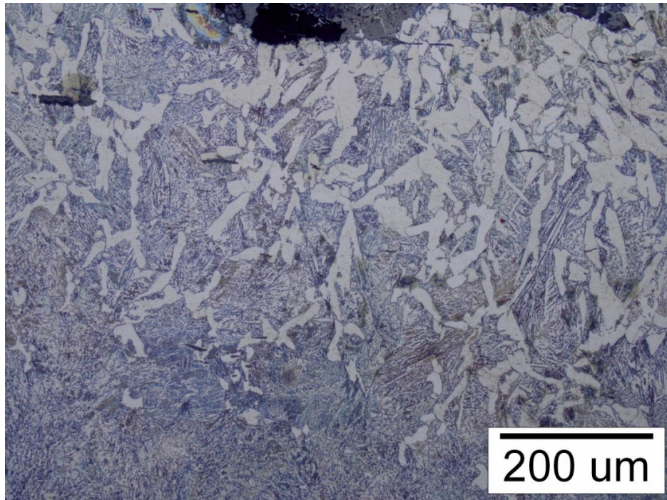
Slika 58. Mikrostruktura na poziciji 6
