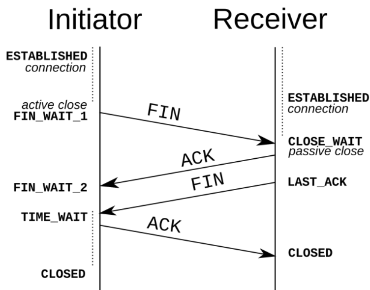
Slika 2.5: „Three-way handshake“
